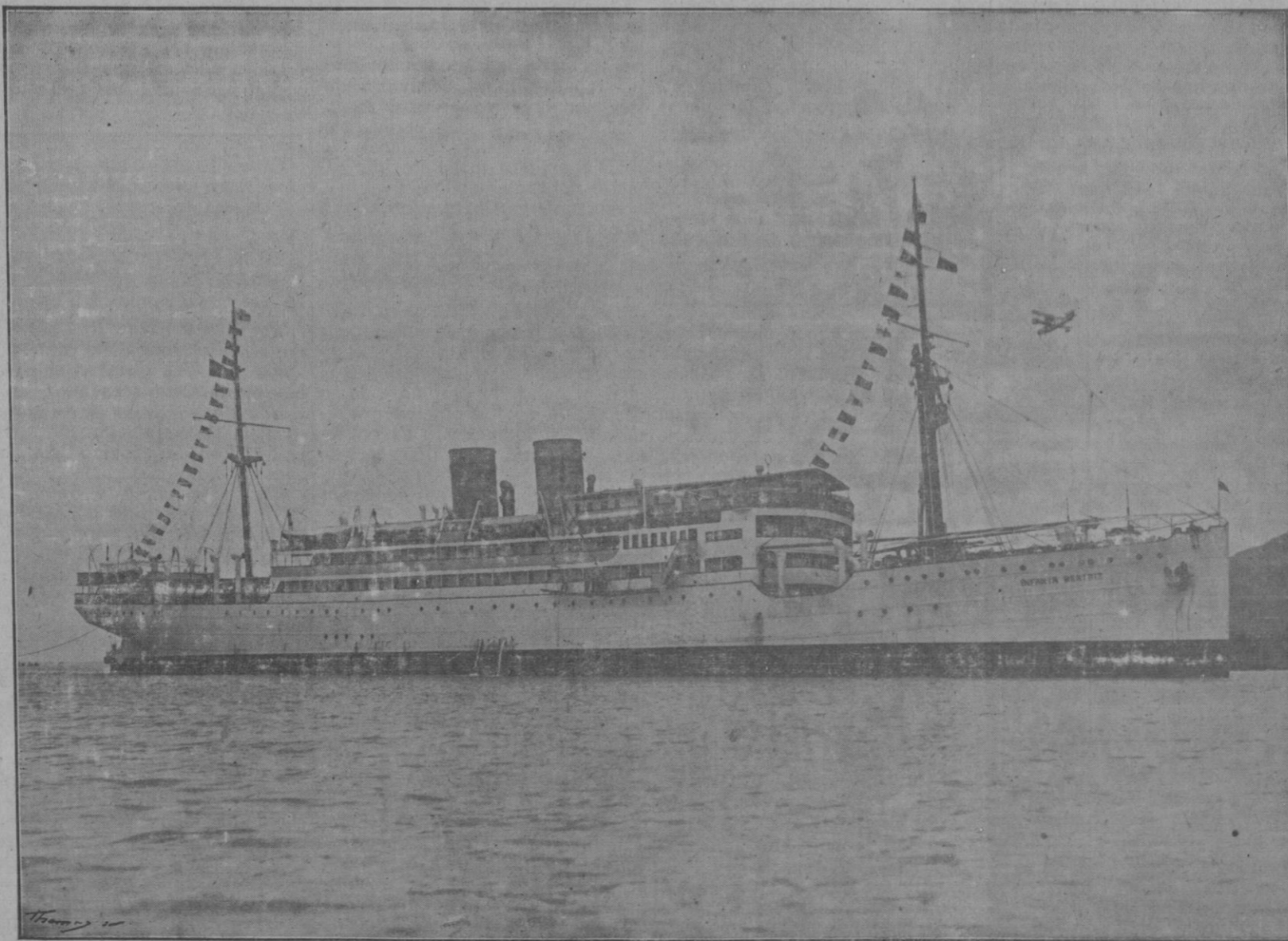
El buque a motor «Infanta Beatriz» recientemente construido por la Trasmediterránea de 9.515 toneladas y 16 millas de andar, cuyas pruebas oficiales se verifican hoy en Barcelona
