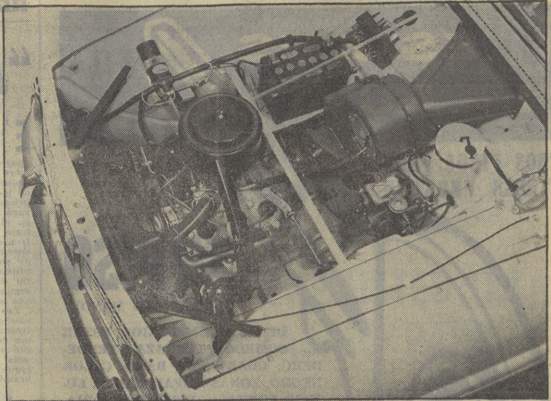
El radiador y la carcasa envuelven perfectamente al ventilador, con lo cual aumenta su eficacia.
