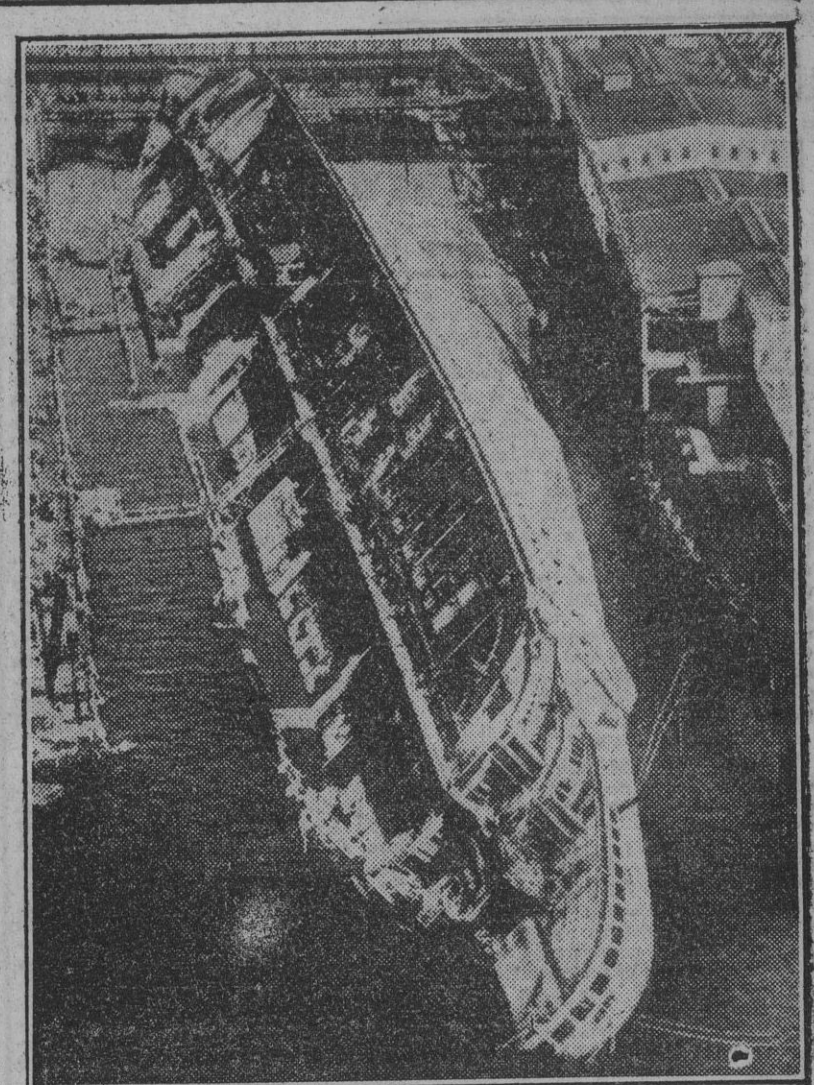
Después de hundido, comenzaron los trabajos para poner el buque a flote. He aquí una vista del antiguo "Normandie", tomada después de varias semanas de trabajo. (Foto A.)
