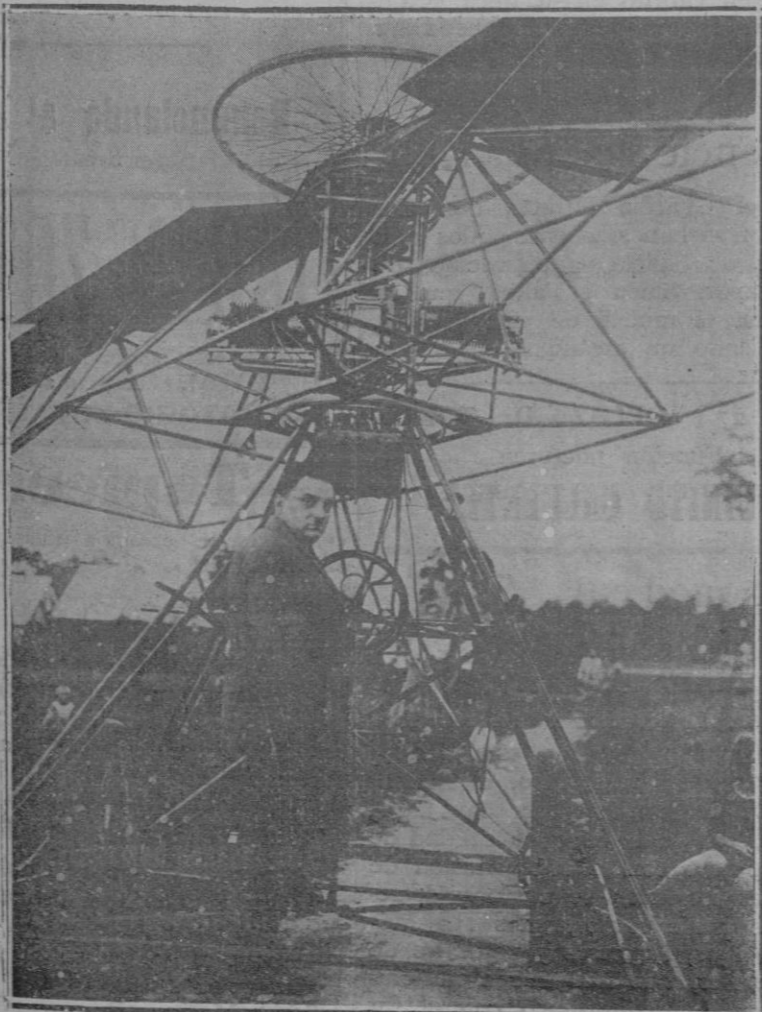
El ingeniero alemán Zaschka, con el helicóptero de su invención, que le permite permanecer parado en el aire y descender verticalmente
