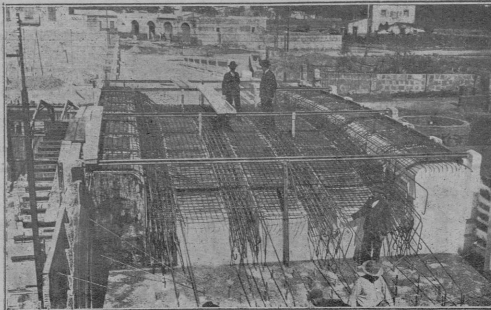
Armado y encofrados del arco en cuya terminación trabajarán mañana más de cien operarios
