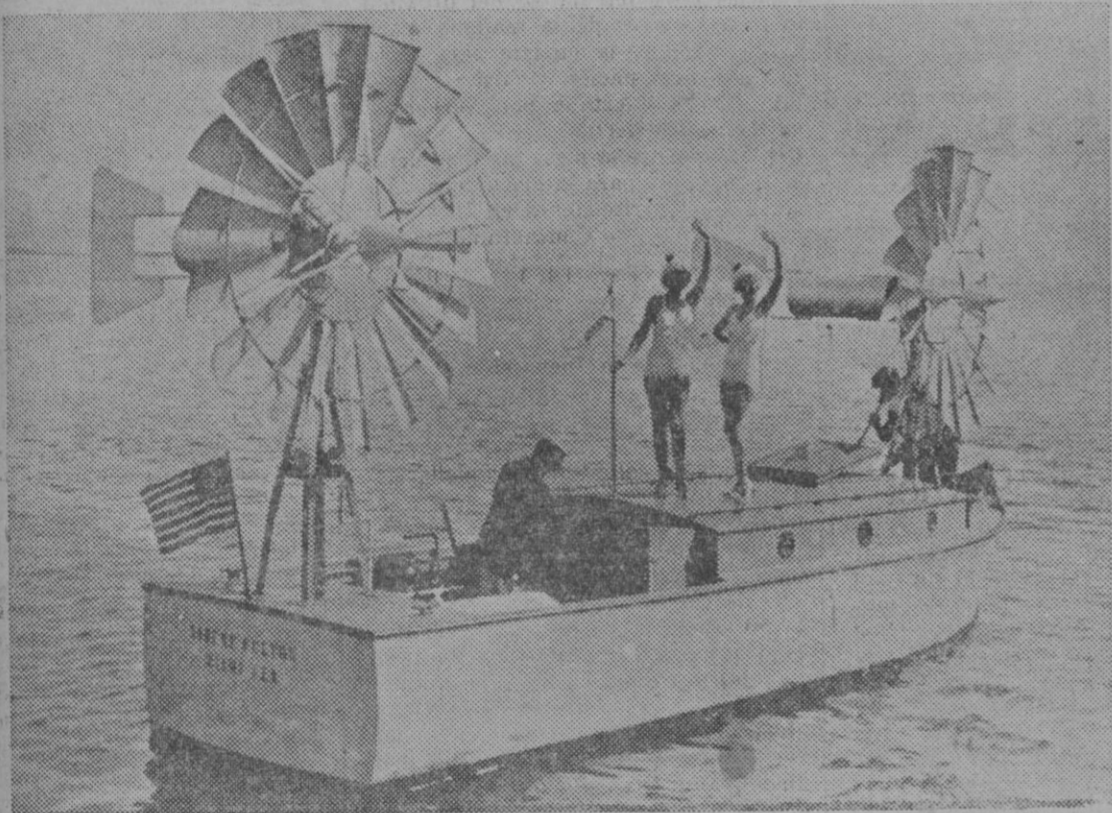
El constructor americano Palmer H. Cray, ha construido su propio bote que utiliza para su movimiento aire comprimido. Los molinos de viento comprimen el aire en un tanque que luego mueve el bote a gran velocidad. El modernísimo bote «Robert Fulton» efectuando pruebas en Miami (Florida). Express-Foto.
