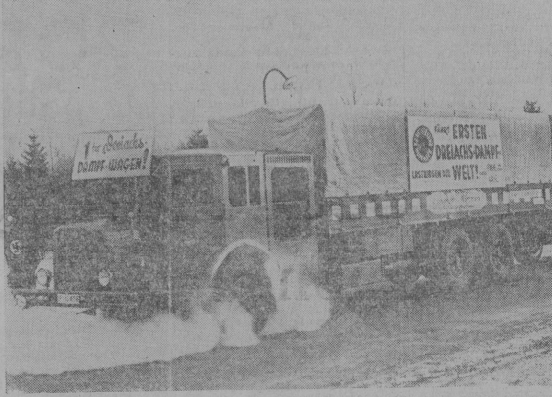
EL PRIMER CAMION A VAPOR DE TRIPLE EJE. — Con objeto de evitar en lo posible la importación de carburantes extranjeros ha sido construido en Hamburgo con buen éxito un camión de tres ejes que emplea como carburante un derivado de la hulla fácilmente obtenible en Alemania. El camión durante el primer viaje de prueba. (Express Foto).
