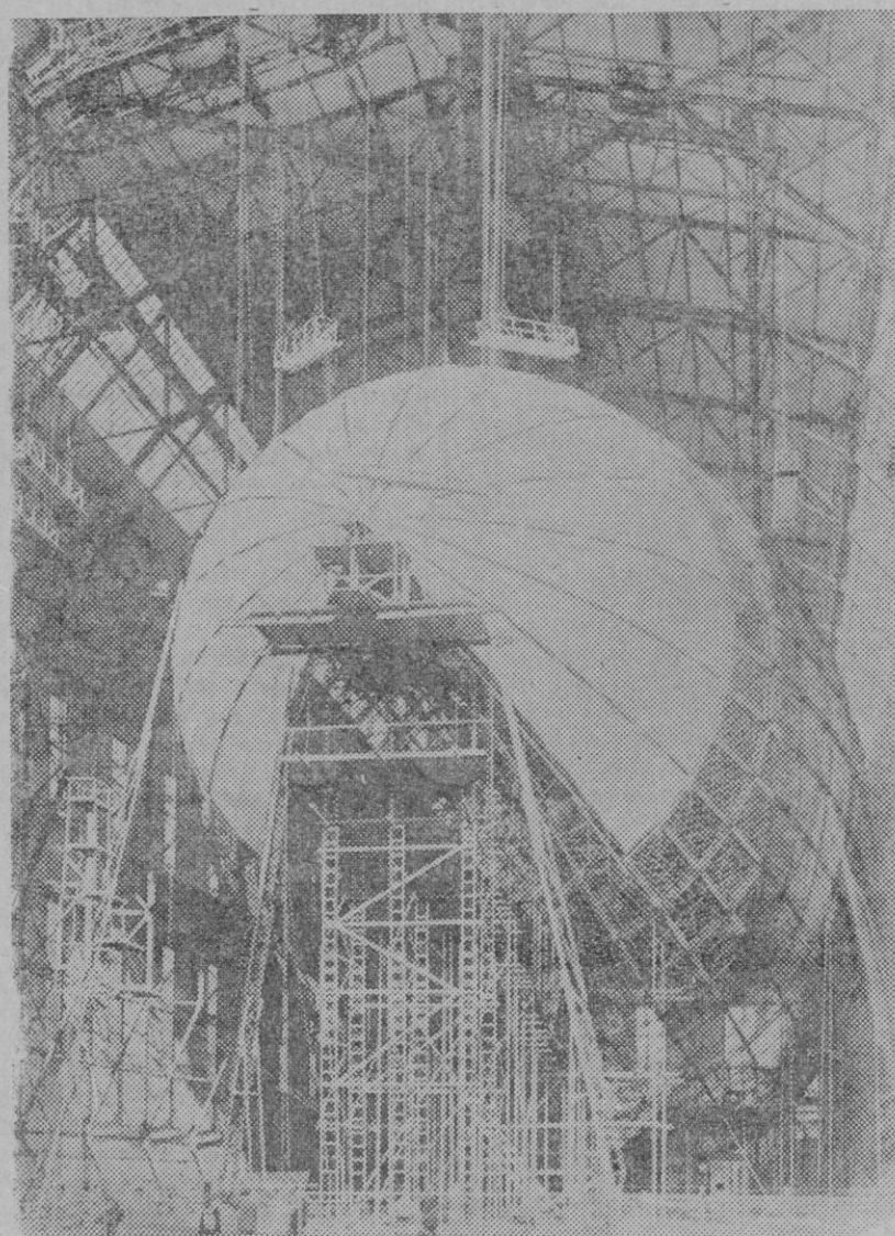
ULTIMA FOTOGRAFIA DE LA CONSTRUCCION DEL LZ 129. — En Friedrichshafen, continúa con gran actividad la construcción del gigantesco Zeppelin LZ 129, al que se está colocando ya la cubierta exterior. Un aspecto de la nave aérea en construcción. (Express Foto).
