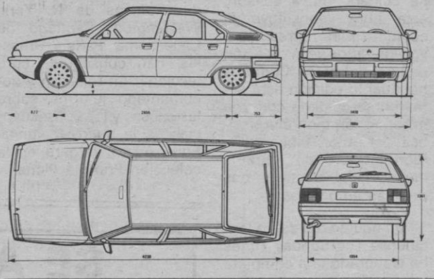
CITROËN BX 16
