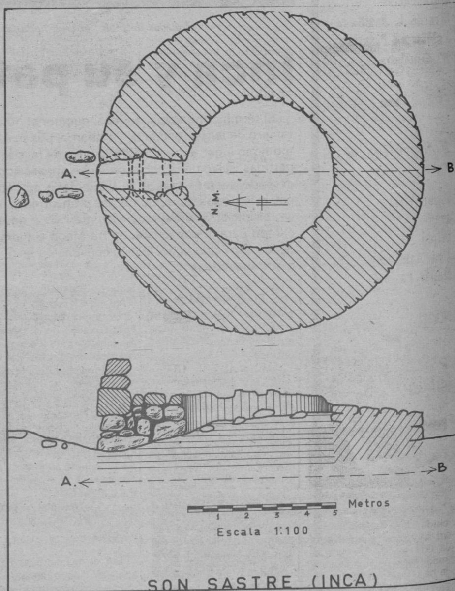
Planta y alzado del talaiot de Son Sastre.
