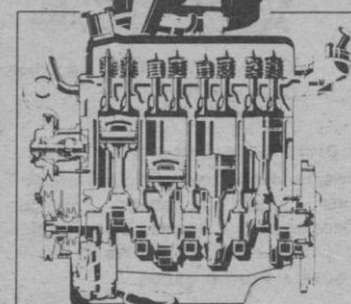
Motor de 1438 cc. y 77 CV DIN
