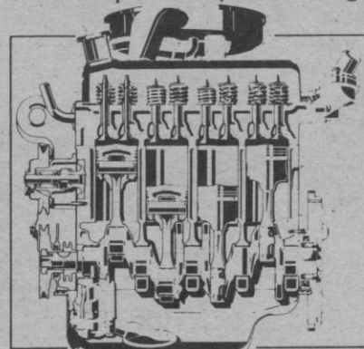
Motor de 1438 cc. y 77 CV DIN
