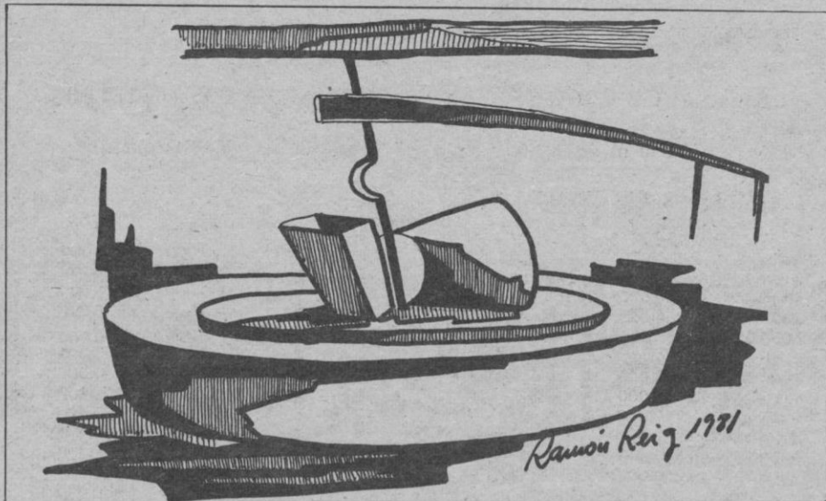
Biga de la tafona de Son Moferes (Calviá) propietat del metge Rotger de Palma, on es pot veure la biga propiament dit, d'una llargari de més de 12 métres, la pila d'esportins i el quintar. Agraint a n'Antoni «Paris», amo d'aquella possessió, el deixarme prendre aquels apunts.
