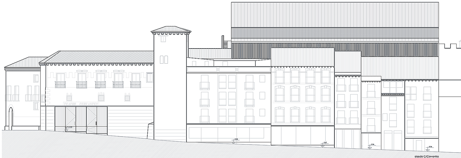
Alzado de la fachada con vistas a la calle Cervantes del proyecto de la UTE Fuster-León-Muñoz-Segovia para la rehabilitación del Teatro Cervantes de Segovia
