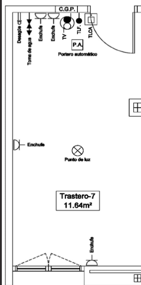
PLANTA SEMISOTANO
