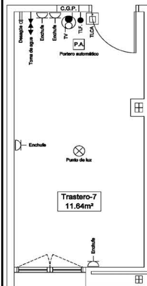
PLANTA SEMISOTANO
