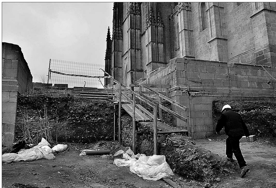
Los trabajos en el talud ya han comenzado con la limpieza y el planteamiento de las obras a realizar. / ALBERTO BENAVENTE
