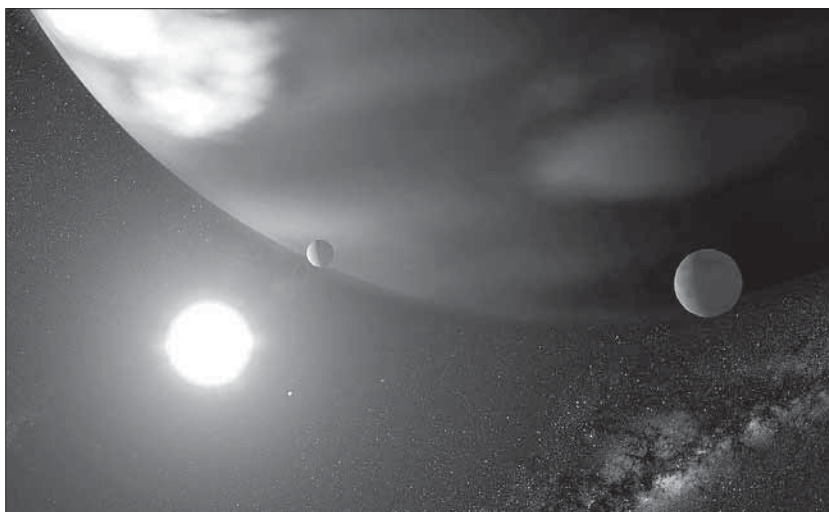
Imagen de la Vía Láctea, donde el astrónomo norteamericano Andrew Gould ha descubierto dos nuevos planetas. / LT
