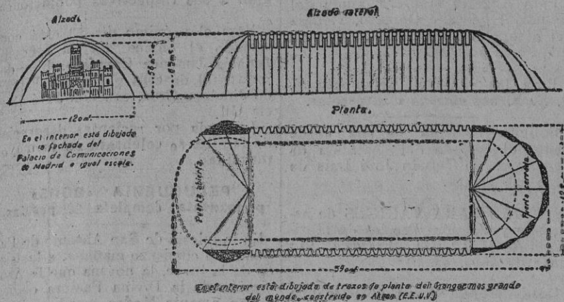
Hangar de hormigón armado para el aeropuerto de Sevilla
