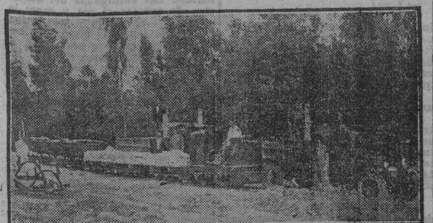
El pequeño ferrocarril para transporte de materiales, tirado por locomotora a gasolina, y camiones utiliza dos en los trabajos del aeropuerto. (Foto. S. del Pando.)
