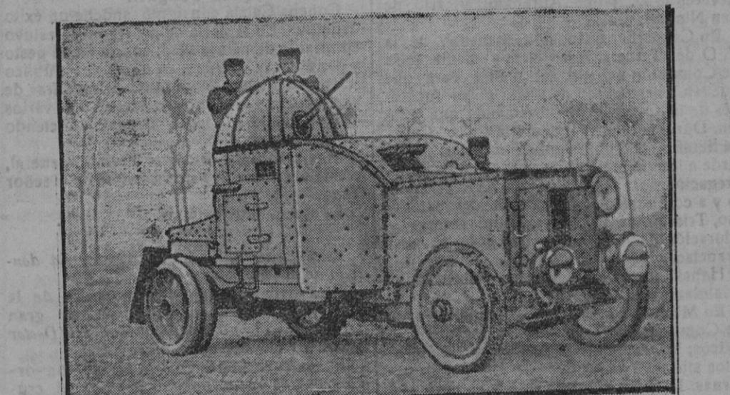
Automóvil blindado, con ametralladoras, perteneciente al ejército francés
