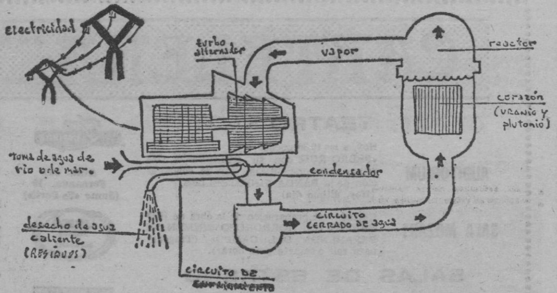
esquema de una central nuclear de agua ligera (CLÁSICA)
