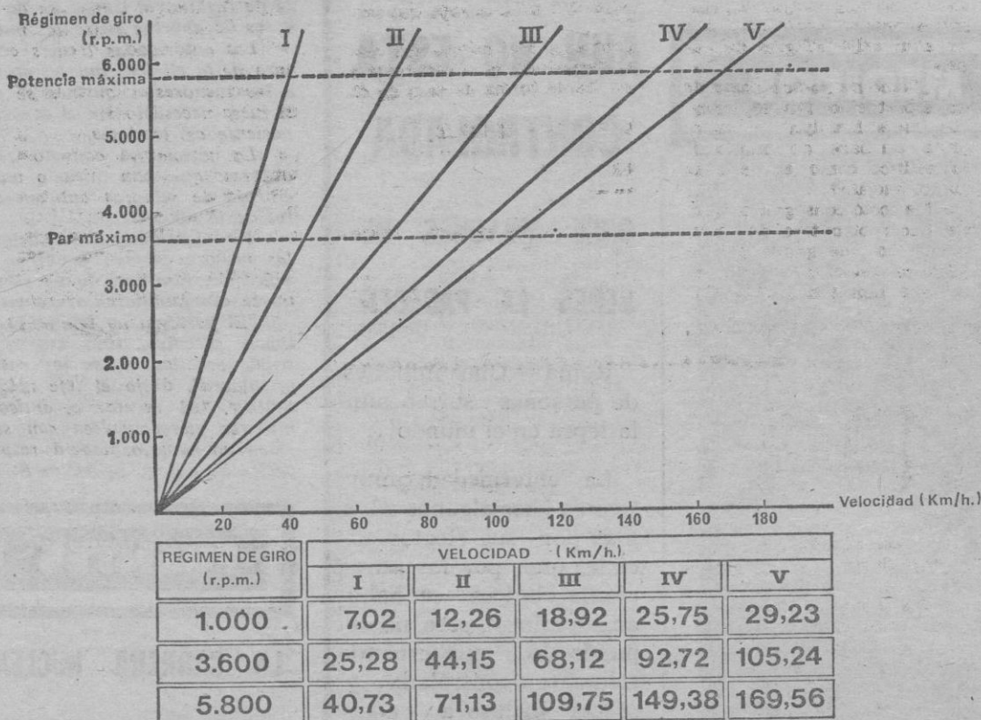
DIAGRAMA DE VELOCIDADES: SEAT 124 D ESPECIAL 1600 (90 octanos)
