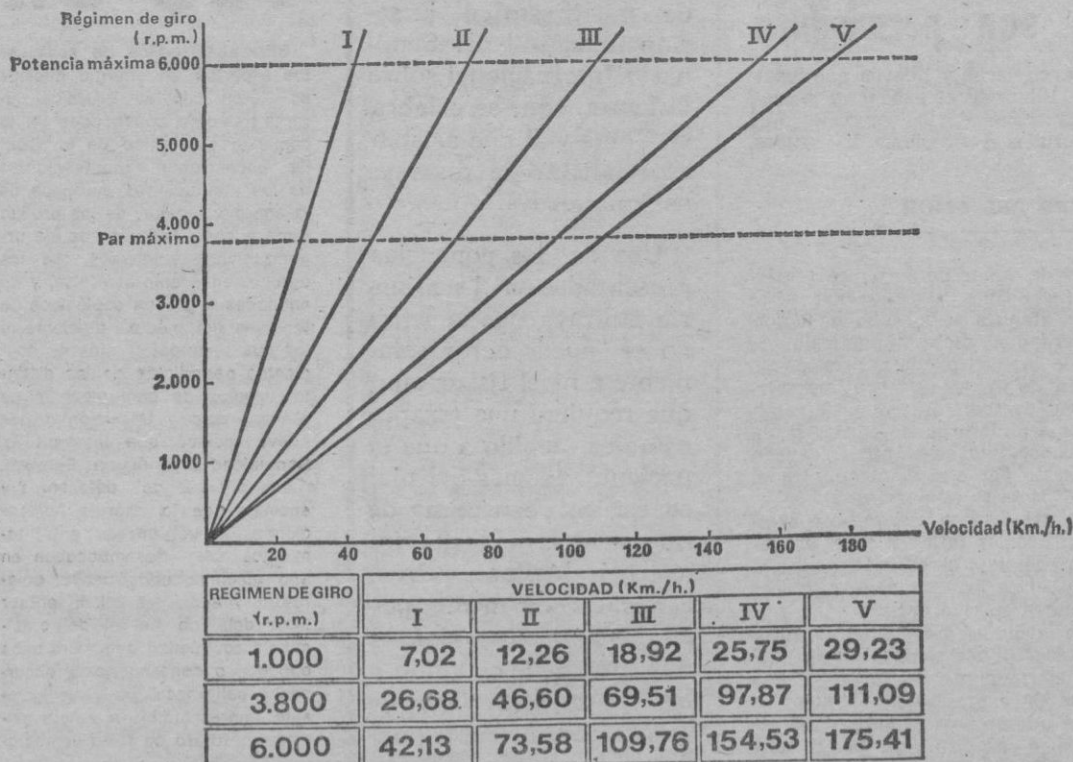
DIAGRAMA DE VELOCIDADES: SEAT 124 D ESPECIAL 1600 (96 octanos)
