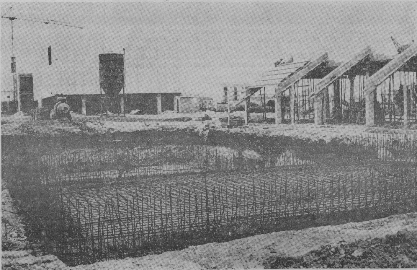
Avanzado estado de las obras de la piscina que se está construyendo, en el Parque Municipal. Al fondo, el teatro que está realizando el Ayuntamiento. Esta piscina es de 25 metros, con tribunas y todas las instalaciones complementarias, como vestuarios, etc.
