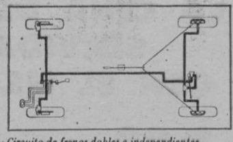
Circuito de frenos dobles e independientes. Corrector de frenada sobre las ruedas posteriores.
