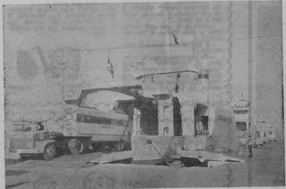
Vehículo especial de TRAFRUME para carga congelada.
