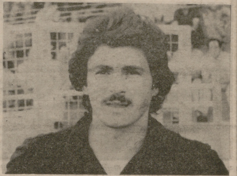
BEBICH
