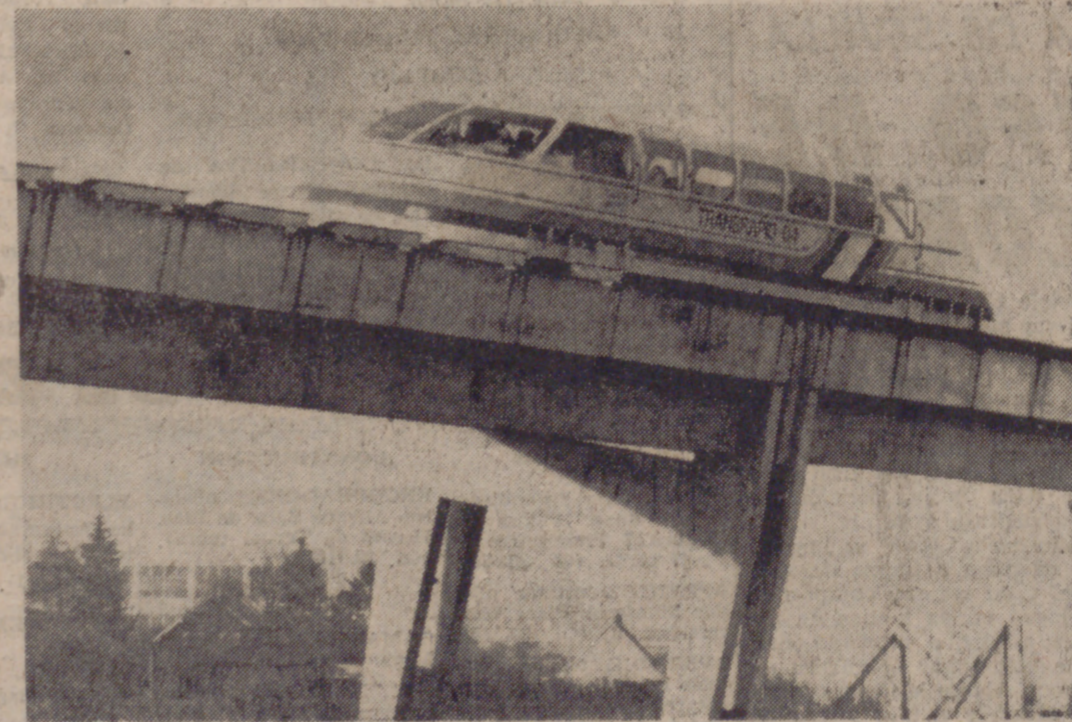
MUNICH (DaD).—Los técnicos alemanes llevan notable ventaja a otros países en la carrera para conseguir el tren del futuro. En la fotografía aparece la locomotora «Transrapid 04», propulsada por un motor eléctrico lineal y que se desliza sobre campos magnéticos. Pesa 16,5 toneladas, alcanza 200 kilómetros a la hora y ha sido concebida conjuntamente por los ingenieros de las industrias Krauss y Maffei. Actualmente esta siendo probada en un circuito experimental de 2,4 kilómetros de longitud situado en las cercanías de Munich.
