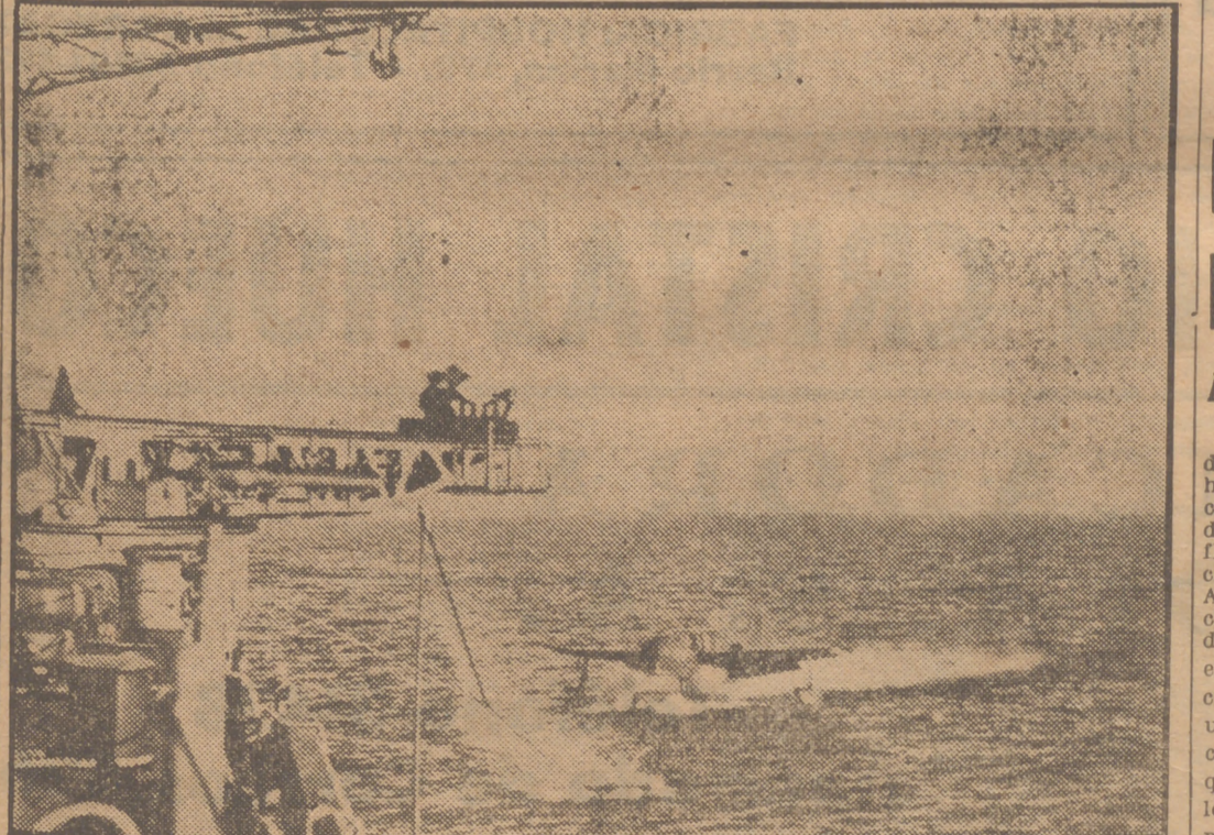
con un avion despegado por la catapulta del "Denver" se verificaron pruebas de un nuevo ingenio para recoger los aparatos de reconocimiento forzados en el mar tras su servicio. Consiste en una red deslizante, sobre la que queda retenido el avión, que es llevado así, sin desviación posible de rumbo, hasta el costado del barco nodriza. Después es elevado por la grúa. (Foto A. P.)
