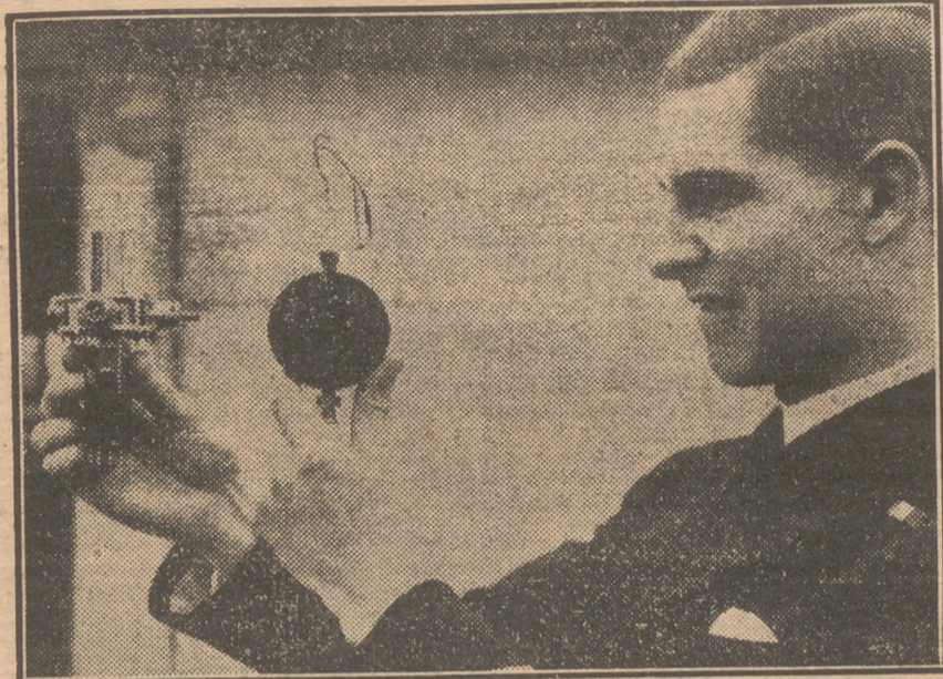
He aquí las válvulas de recepción y de transmisión usadas en los equipos de "radar". A la izquierda, la válvula de transmisión Magnétron, y a la derecha, la válvula de recepción Sutton. (Foto Cifra.)
