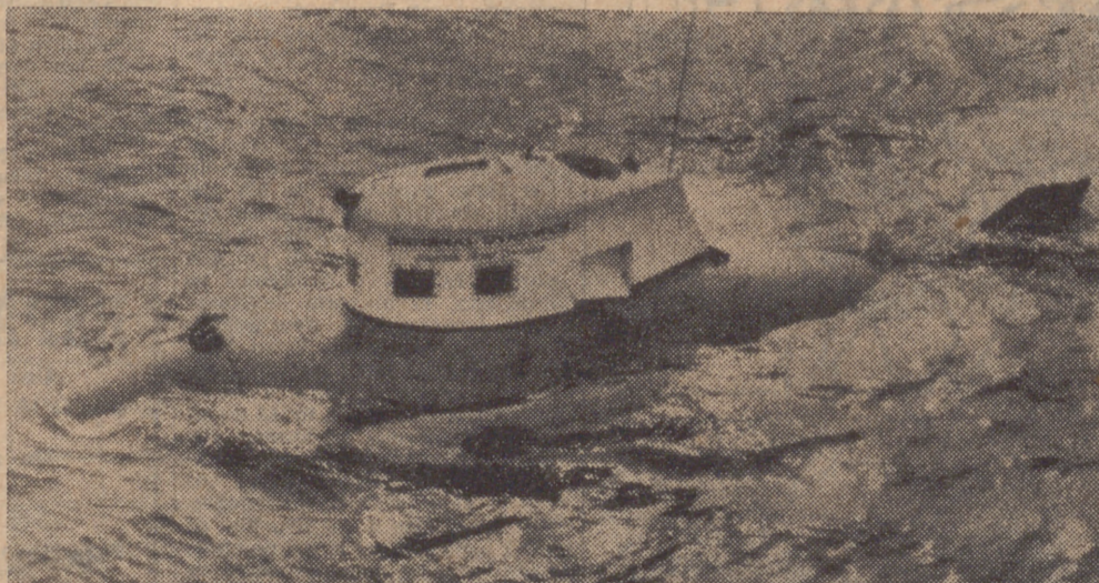
Un submarino de dos plazas utilizado para explorar el fondo del mar, el «Star III», construido por la General Dynamics, de Connecticut. Un brazo mecánico de proa está diseñado para cortar alambres, otro para coger conchas y una «mano» que puede coger tanto un lápiz como un objeto de 90 kilos
