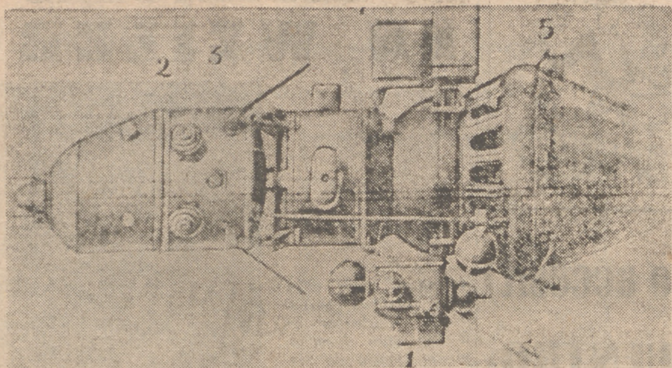
El periódico "Pravda" publicó este dibujo explicativo del "Luna X", puesto en órbita lunar por Rusia: 1) Radio. 2) "Sputnik" lunar. 3) Sistema de separación del "Sputnik". 4) Equipo de astro-orientación.
