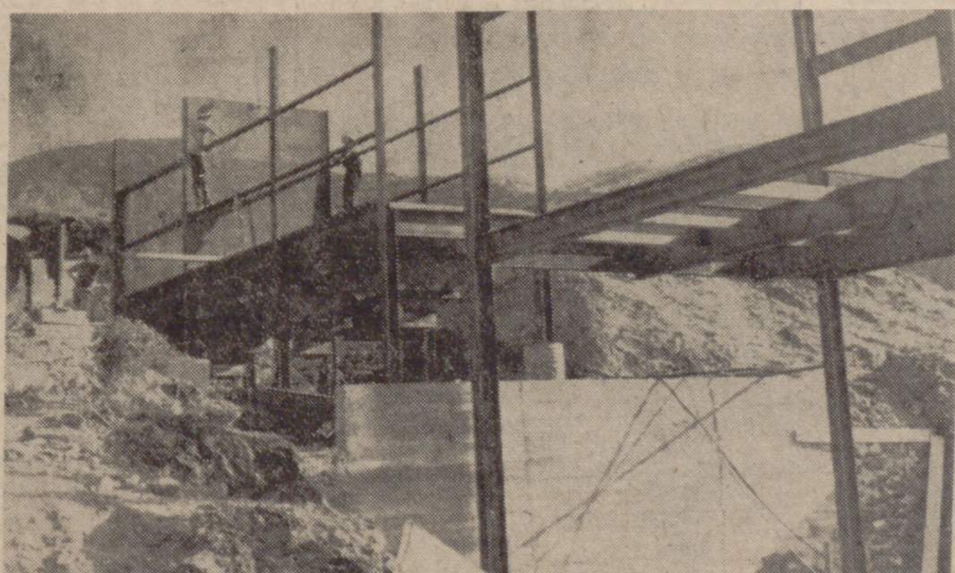
CARRATRACA (Málaga).—Treinta hombres trabajan en el montaje de la planta piloto en la mina "Teync", amén de los técnicos de la Compañía Asturiana de Minas, para la búsqueda de diamantes en esta zona malagueña. Diariamente llega maquinaria y se espera que las instalaciones necesarias queden terminadas el día 15 de julio.—(Foto Cifra Gráfica.)
