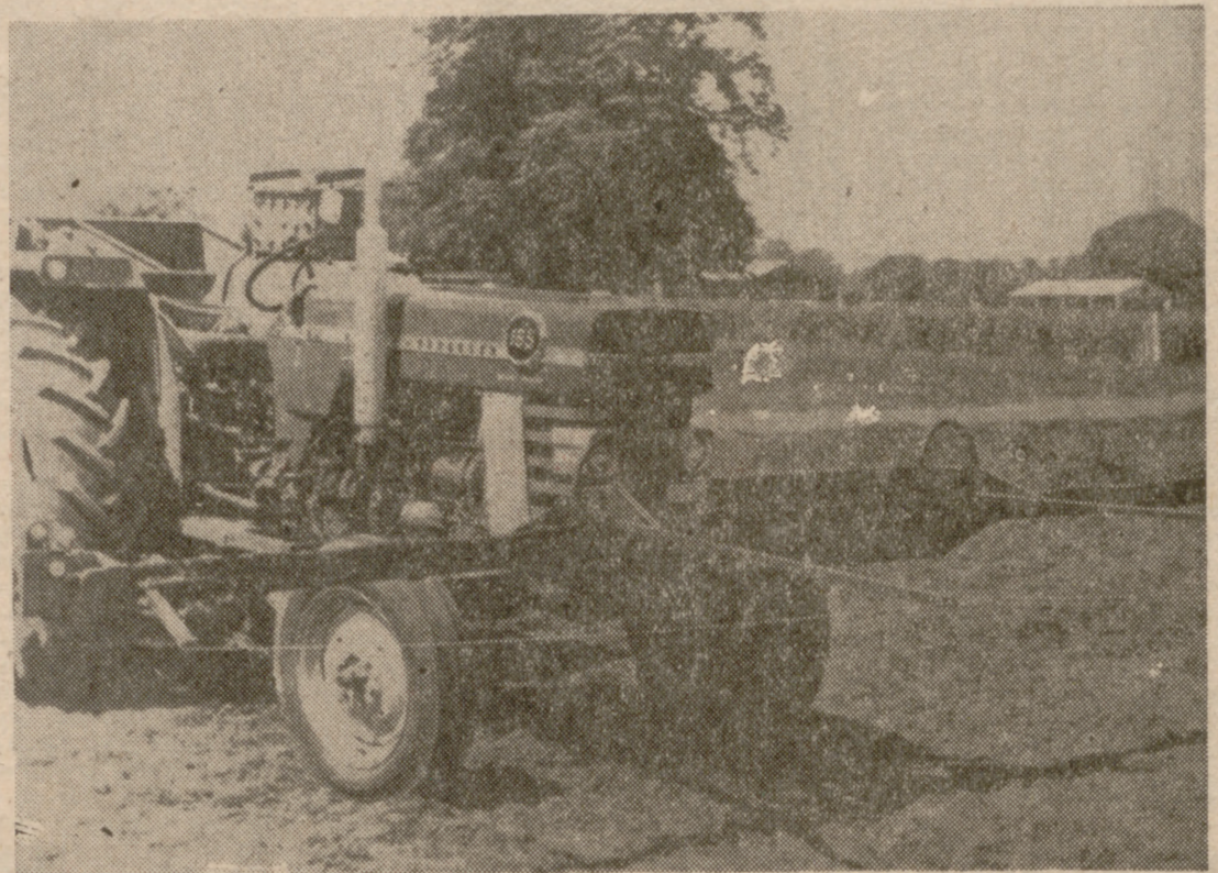
Un tractor, equipado con uno de los sistemas que se tratan en el presente artículo, que puede realizar toda suerte de trabajos agrícolas sin necesidad de conductor.
