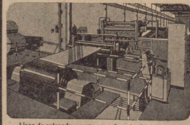
Línea de aplanado y corte para chapa laminada en caliente. Anchura máxima 2 m. Espesor de 1'5 a 7 m/m. Largo máximo 11 m.
