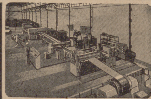
Línea de corte longitudinal para flejes en cualquier ancho hasta 1500 m/m. partiendo de bobinas laminadas en caliente y en frío.
