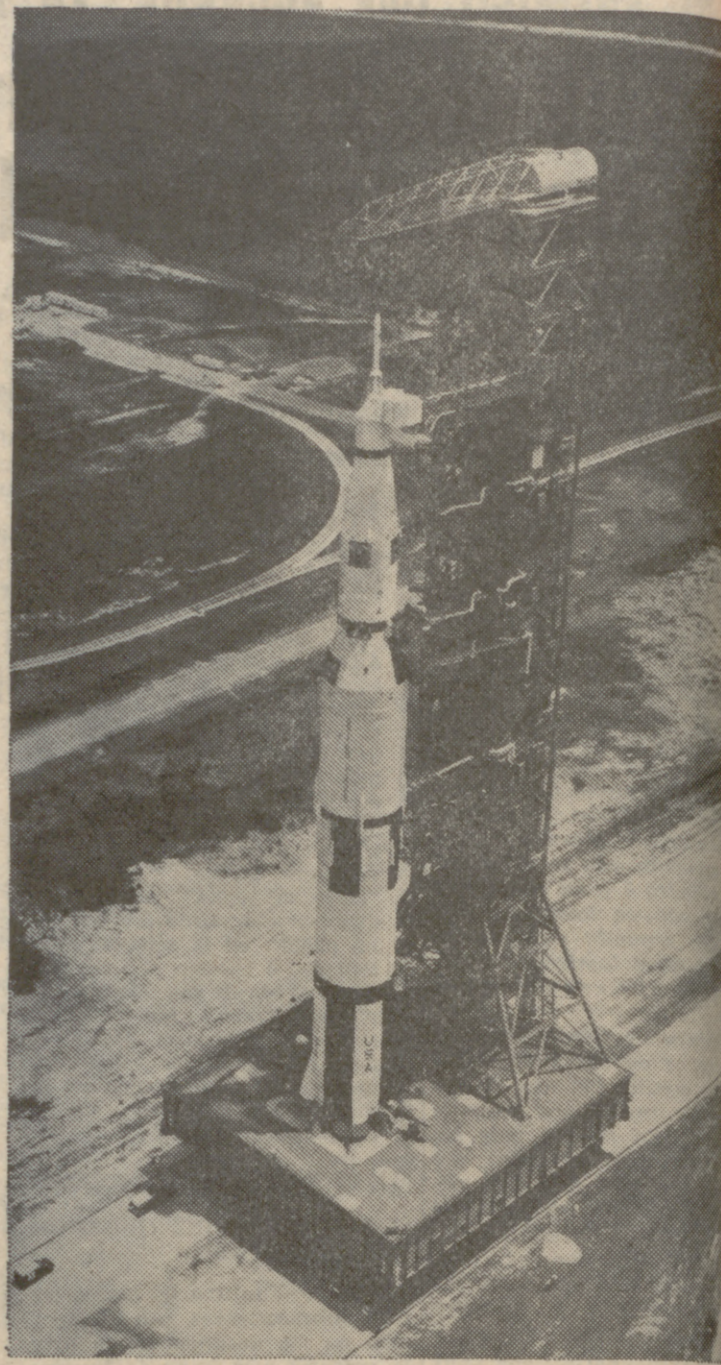
Modelo del cohete "Saturno V" que lanzará a la Luna una astronave con tres astronautas norteamericanos a fines de esta década, es trasladado desde el edificio vertical de ensamblaje a la plataforma de lanzamiento en Cabo Kennedy (Florida). El cohete, de 111 metros de alto, es conducido por una gigantesca grúa de 3.000 toneladas.
