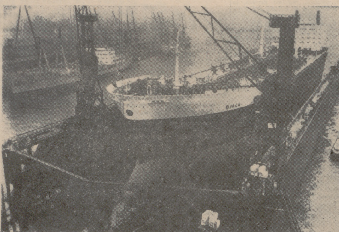
En lo sucesivo podrán repasar y repasar en la República Federal de Alemania también superpetroleros. El dique flotante más grande de Alemania y uno de los más potentes en toda Europa, acaba de ponerse en servicio en el puerto de Hamburgo. El "Dique flotante 7", de 253 m. de largo y 53 m. de ancho, acusa una potencia elevadora de 47.000 toneladas.
