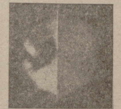
Imágenes del Planeta con luz ultravioleta e infrarroja. Se han juxtapuesto las imágenes contrarias de las dos imágenes para mostrar que la imagen a la luz ultravioleta es mayor. La imagen a la luz infrarroja, que muestra los detalles superficiales, representa el globo sólido; la ultravioleta, en la que no se distingue ningún detalle superficial, representa el globo sólido rodeado por la envoltura atmosférica.
