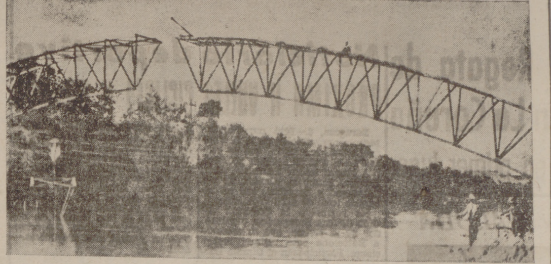
Un momento emocionante de la construcción del puente de El Cubo, sobre el Pisuegra; el encuentro de las cimbras metálicas, a punto de acordarse. ¿Falta poco, verdad? De la emoción de los técnicos participa el público en estos días. Cientos de personas contemplaron ayer la colocación de los elementos del cimbraje. El espectáculo resulta entretenido, instructivo y muy barato. — (Foto CARVAJAL.)
