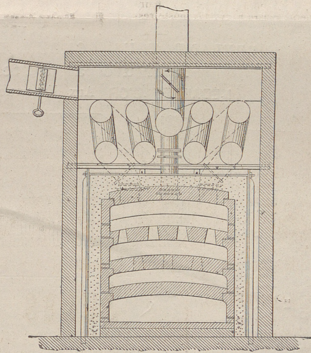
Fig. 2 Coupe transversale
