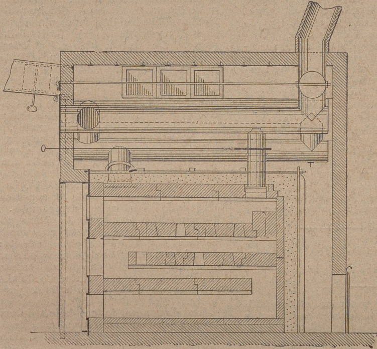
Fig. 1 - Coupe longitudinale
