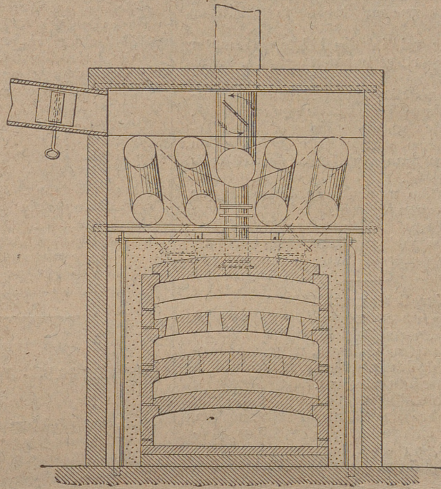
Fig. 2 - Coupe transversale
