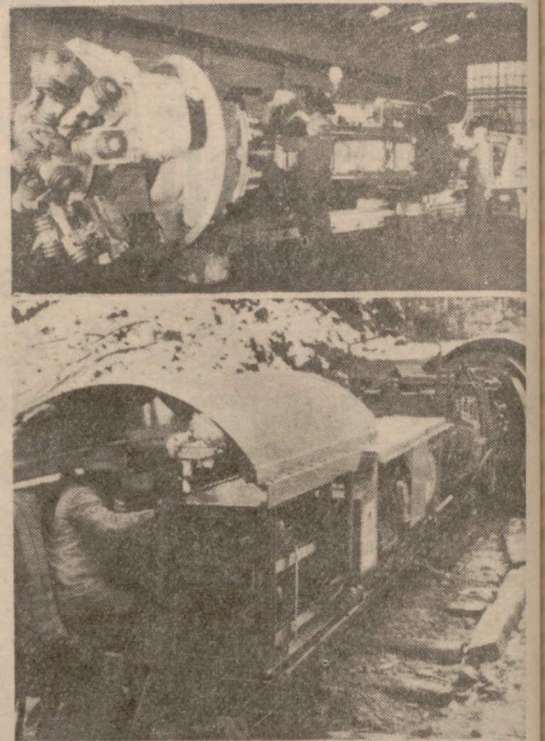
Este "topo de acero" despedaza con su cabezal portablocas, y con una presión de cien toneladas, piedras diez veces más duras que el hormigón armado. Nuestra foto hace ver la máquina en la construcción de una cañería para agua potable, que en parte pasará 50 metros debajo de la superficie del terreno y a través de rocas de una resistencia de 800 hasta más de 2.000 kp/cm 2 . No obstante, la perforadora avanza con una velocidad de casi dos metros por hora. En la construcción de túneles se puede alcanzar mediante ella un ahorro de tiempo del 50 por 100. La máquina es maniobrada por un solo conductor. Su marcha es vigilada de modo enteramente automático. Un rayo Laser de color marca el eje del túnel.
