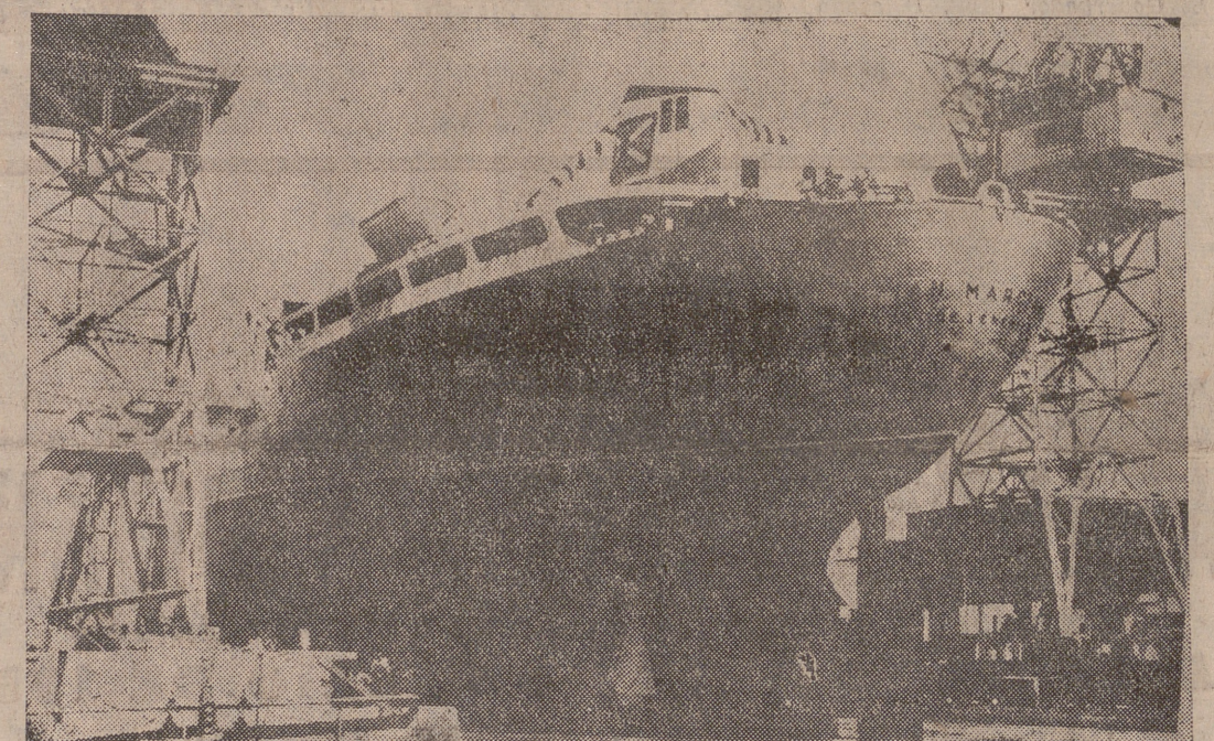
Cádiz.—Momento de la botadura del nuevo buque tanque "San Marcial" en los astilleros Matagorda, de la Sociedad Española de Construcciones. Dicho barco, gemelo del "Talavera", desplaza 42.250 toneladas, con una velocidad en pruebas de 17 nudos, y va dotado de turbinas "Parsons" de 14.000 caballos a 105 revoluciones por minuto. Presidió el acto el ministro de Hacienda, señor Navarro Rubio. (Foto Cifra Gráfica)
