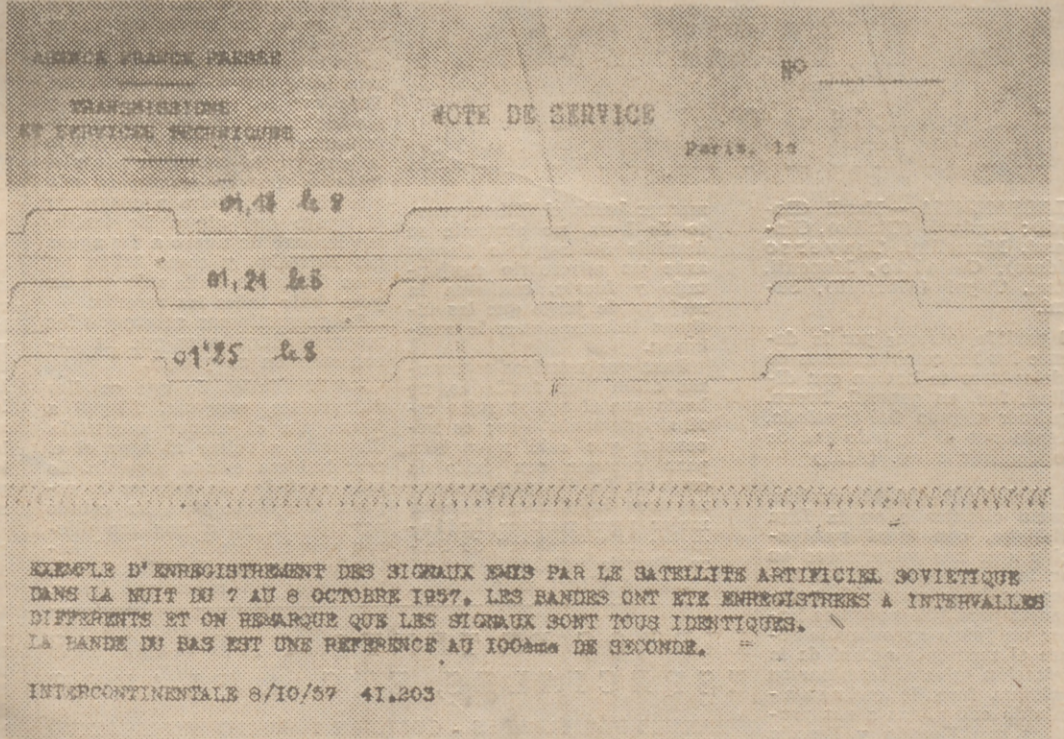
Este es un ejemplo del registro de las señales emitidas por el satélite artificial ruso en la noche del 7 al 8 de octubre. Las bandas están registradas a intervalos diferentes, y obsérvese cómo todas son idénticas. La banda inferior es una referencia de una centésima de segundo.
