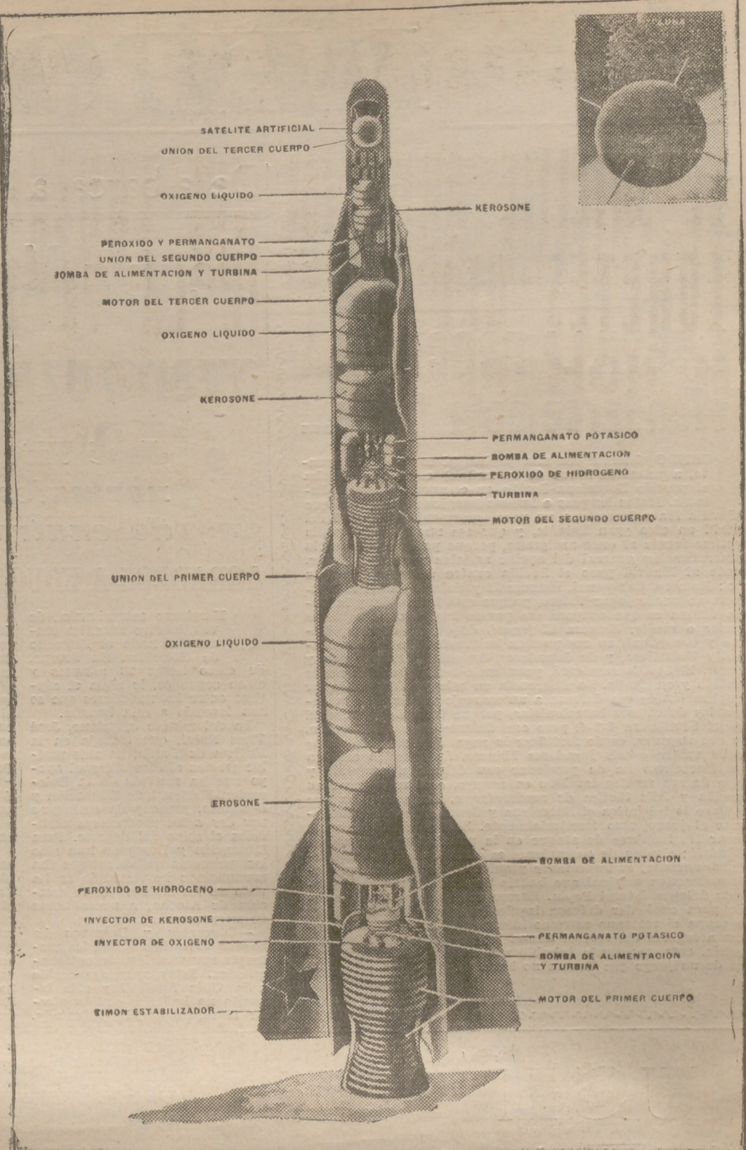
Este es exactamente el contenido del cohete portador del satélite artificial ruso. En el gráfico puede apreciarse el contenido de los proyectiles que conducen al satélite hasta su órbita
