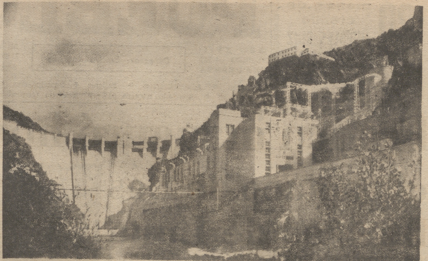
Una vista de la presa y de la central hidroeléctrica de San Esteban del Sil, que acaban de ser inauguradas por el Jefe del Estado. (Foto Cifra)
