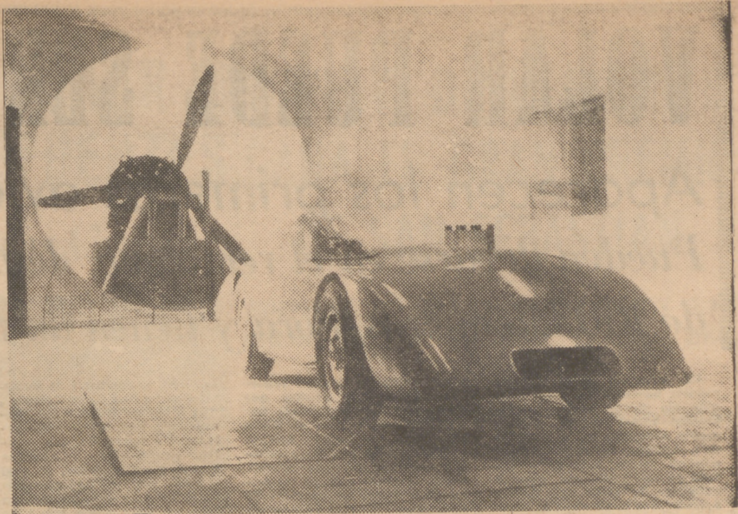
Este coche Austin, conducido por Donald Healey, ha superado 28 records internacionales en Bonneville, a una velocidad de 203 millas por hora. Este "carro" está equipado con una capota que se cierra automáticamente, con carrocería especial adaptada a su singular condición de "tragami-llas" y con un motor que marcha a 5.000 revoluciones. Es una máquina portentosa, que corre a velocidades de avión. Si no llevase la cabina cerrada, el conductor no podría resistir tal presión del aire.
