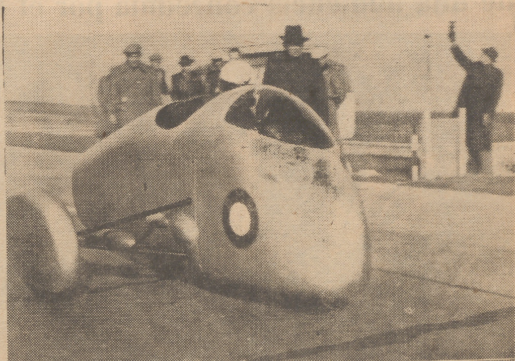
Wilhelm Noll, sobre su máquina B. M. W., al tomar la salida en la autopista de Ingoistad el pasado 23 de noviembre, para batir los records mundiales de los 10 kilómetros y las 10 millas de la categoría sidecars de 500, 750 y 1.200 centímetros cúbicos
