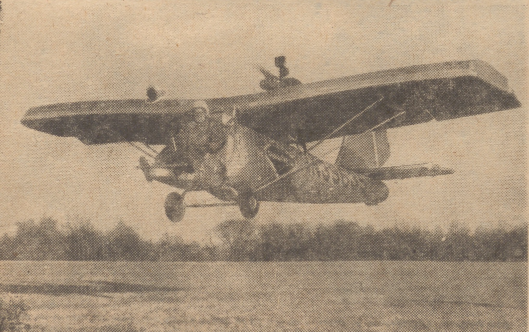
El avión hinchable de la Good Year norteamericana, firma especializada en la construcción de aparatos menos pesados que el aire, fotografiado en vuelos de pruebas
