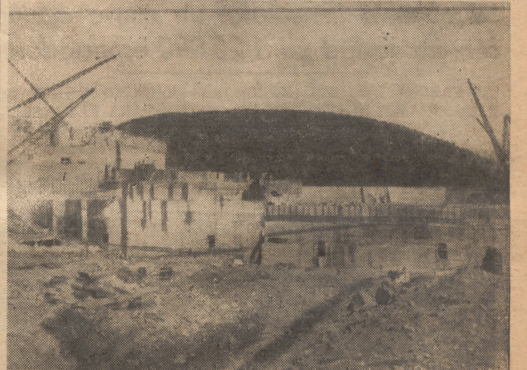
Un aspecto de la presa del pantano Gabriel y Galán, que embalsará más de mil millones de metros cúbicos y que permitirán el riego de una importante zona de la provincia de Cáceres.
