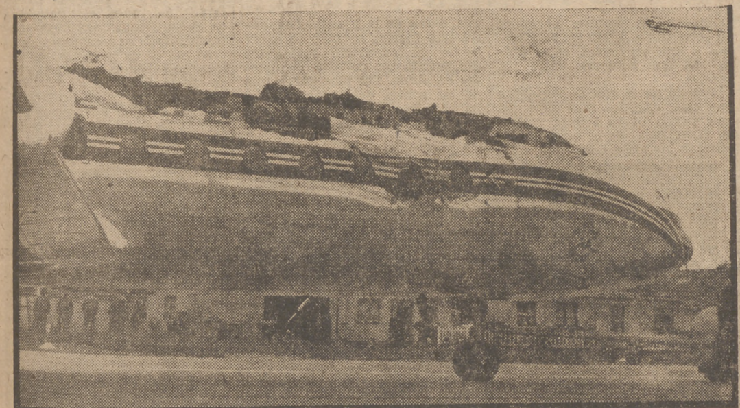
ASI QUEDO EL «CARAVELLE».—Estado en que quedó el avión «Caravelle», de las líneas aéreas argelinas, después del choque con un avión de turismo en el aeropuerto de Orly. Como puede observarse, la parte superior del fuselaje fué totalmente levantada en el choque
