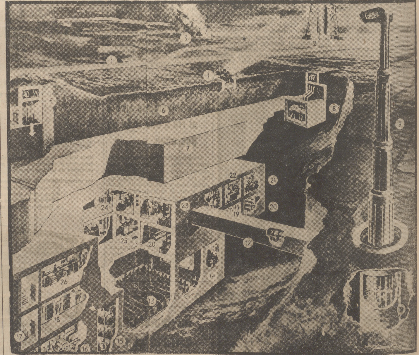
Este es el Cabo Cañaveral ruso, situado en el desierto de Krasnyi Jar. Siguiendo las instrucciones del sueco Larsson, un dibujante ha podido reconstruirlo: 1) La pista para los transportes pesados; 2) Rampa de lanzamiento de proyectiles; 3) Descargas de gas; 4) Reflectores; 5) Entrada al refugio; 6) Capa de terreno de cinco metros; 7) Techo de cemento de cinco metros; 8) Cisterna subterránea y conductos de hidrógeno; 9) Periscopio móvil; 10) Cabeza del periscopio con la cámara de TV.; 11) Motores del periscopio; 12) Cueva del periscopio; 13) Cabina para proyecciones de TV. capaz para trescientas personas; 14) Cabina para el proyector de TV.; 15) Cisterna de agua; 16) Generadores eléctricos; 17) Escalera; 18) Acceso a las habitaciones de estar; 19) Baños; 20) Dormitorios; 21) Puesto de mando; 22) Mando del lanzamiento con transcriptor de cinta; 23) aparato de medida y control
