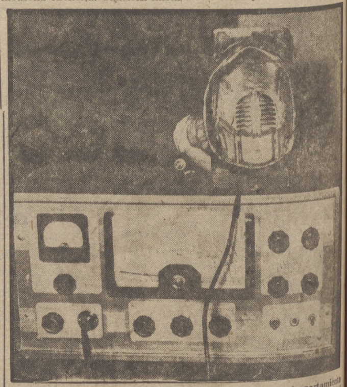
Cuando la Policía de la Hacienda Italiana entró en el apartamento del escritor-contrabandista Pierre-Maurice Chiarena, un oficial encontró en el baño de servicio este aparato radiotransmisor, con el cual se dirigía el tráfico de la mercancía
