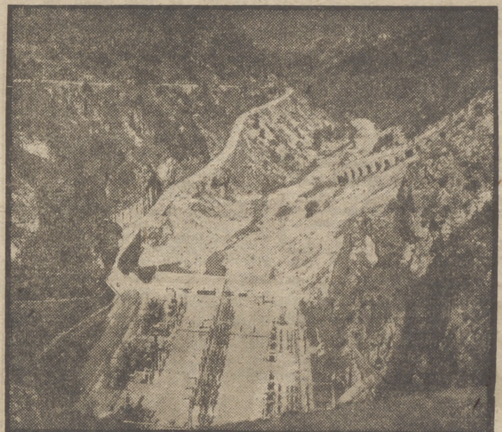
Vista de las instalaciones del pantano del Tranco, capaces para producir cincuenta millones de kilovatios-hora, destinados a la industrialización de Jaén, cuyas obras han sido inspeccionadas por el ministro de Obras Públicas durante su reciente viaje
